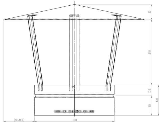
Priemer ( \varnothing D ) od 250 mm
